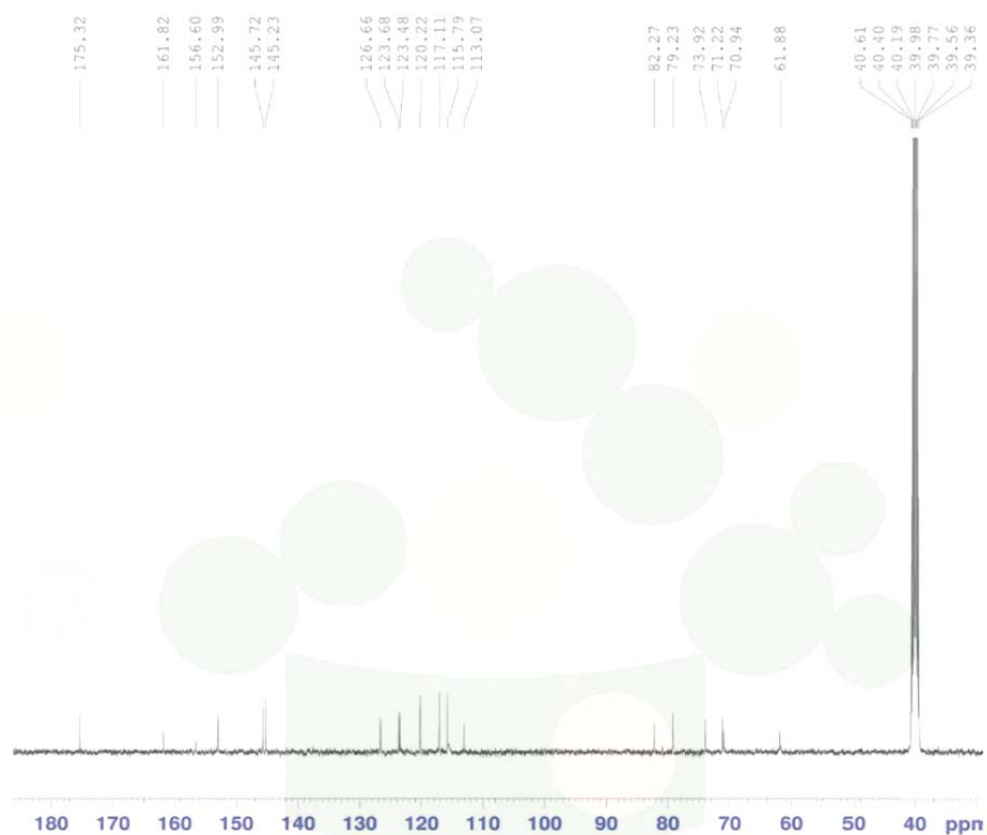
附 3b : ^{13}\text{C} -NMR(100M Hz , DMSO)
